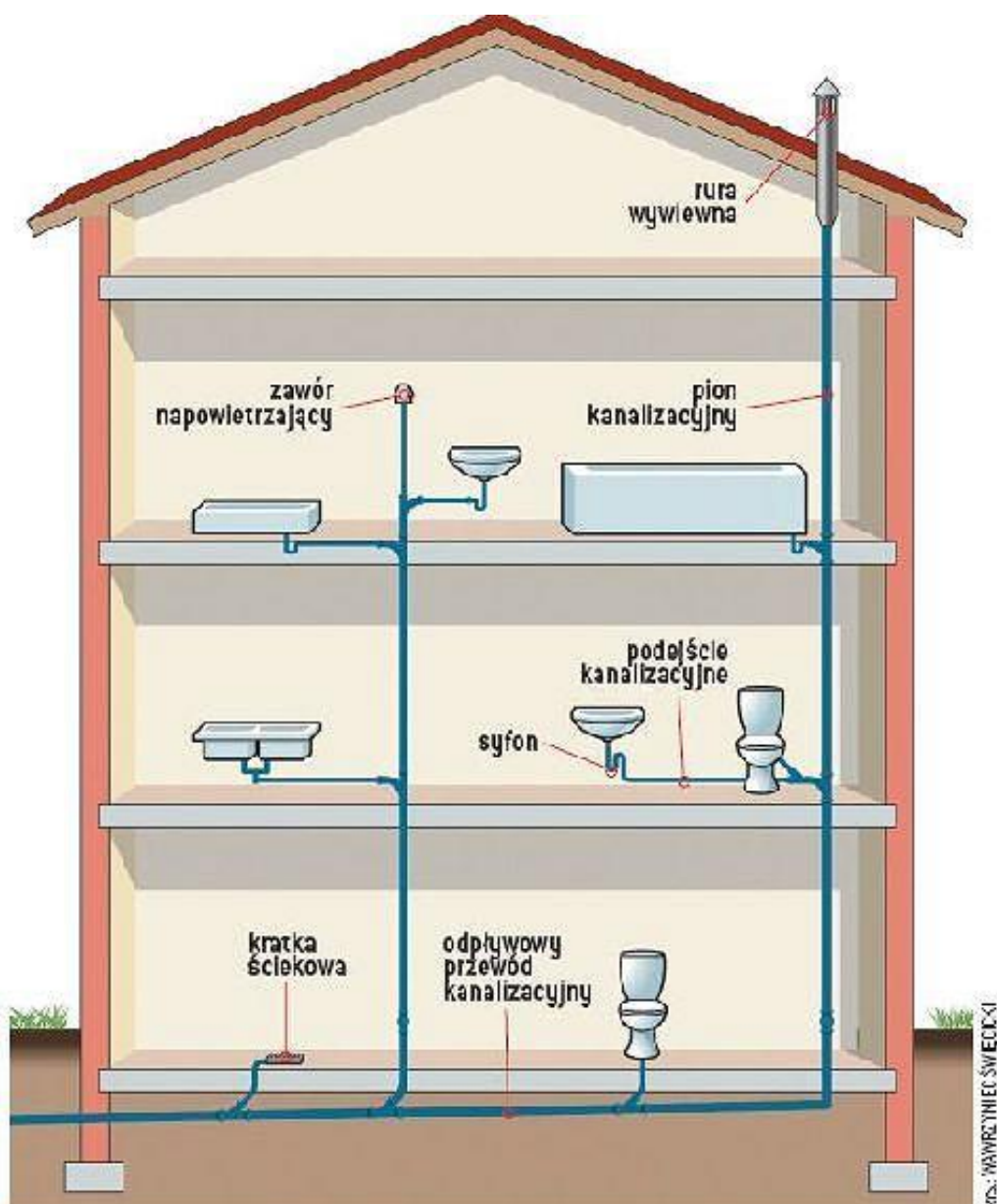
Rys. 1. Rysunek poglądowy – przykład wentylacji instalacji kanalizacyjnej
